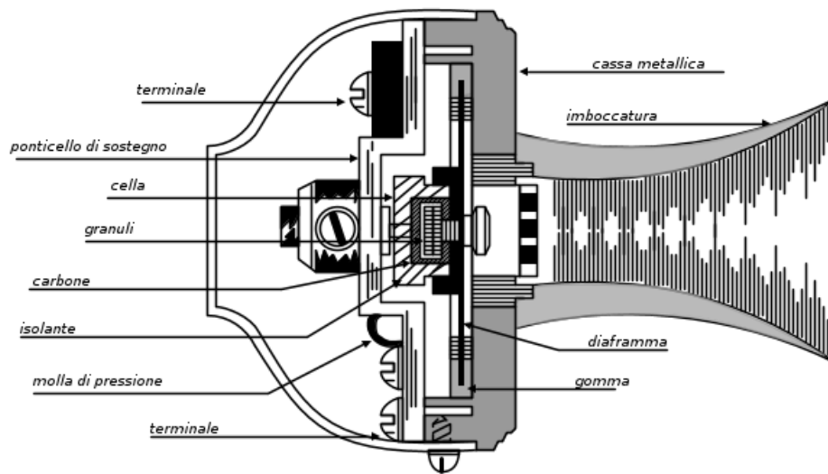
Microfono a granuli di carbone
